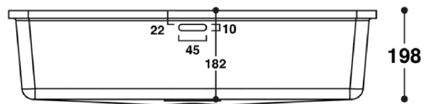
Schnitt-vorne
